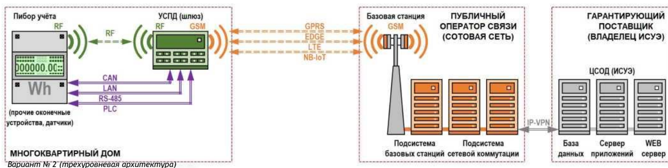
Рисунок № 1 Организация каналов (линий) связи на базе интерфейсов PLC и RF.
